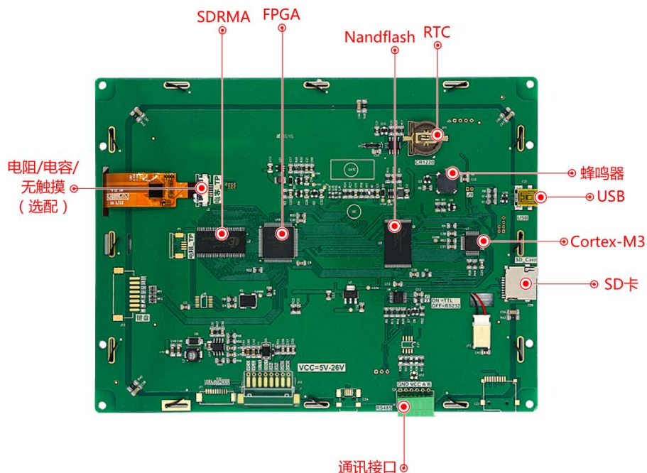
图 1-4 硬件配置图
